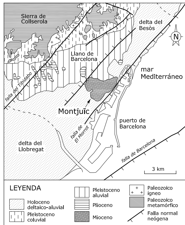
Fig. 1.—Mapa geológico del entorno de Montjuïc, adaptado del ICC (2005). La falla de Barcelona procede del estudio de Bartrina et al. (1992). Las otras fallas proceden del estudio de Llopias Lladó (1942a).
